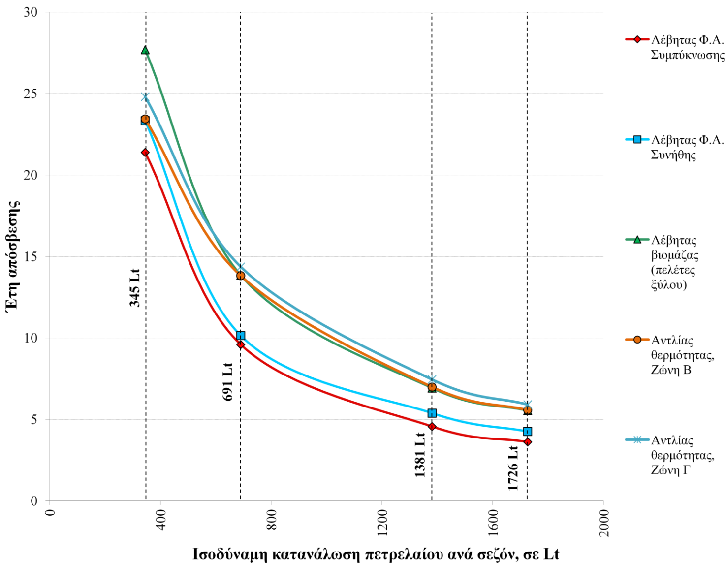
Διάγραμμα 3: Έτη απόσβεσης ανά είδος θερμικού συγκροτήματος για εγκατεστημένη ωφέλιμη θερμική ισχύ 20kW, σε υφιστάμενη εγκατάσταση
