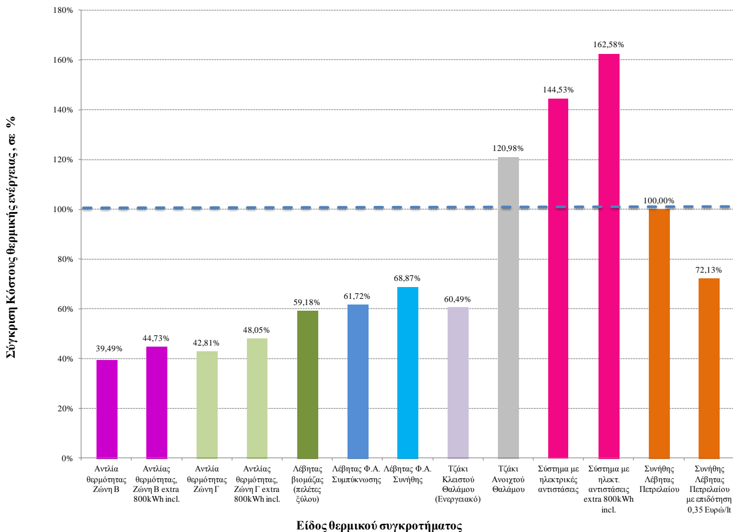
Διάγραμμα 2: Σύγκριση κόστους θερμικής ενέργειας σε %, σε σχέση με το κόστος ενός συγκροτήματος συνήθη λέβητα – καυστήρα πετρελαίου (για τιμή πετρελαίου ~1,256 €/lt), ανά είδος θερμικού συγκροτήματος
